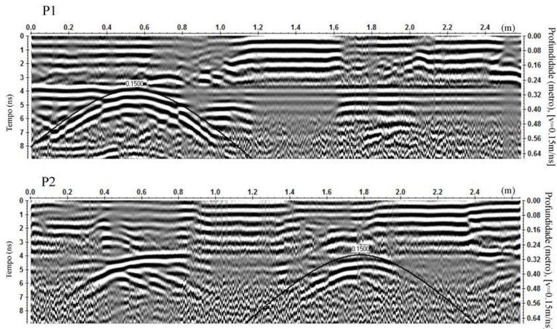
Figura 4: Perfis de georadar P1 e P2 com ajuste de velocidades
