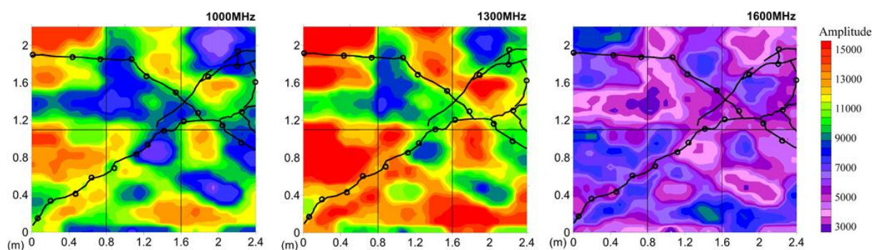
Figura 8: Distribuição de amplitude de frequências
