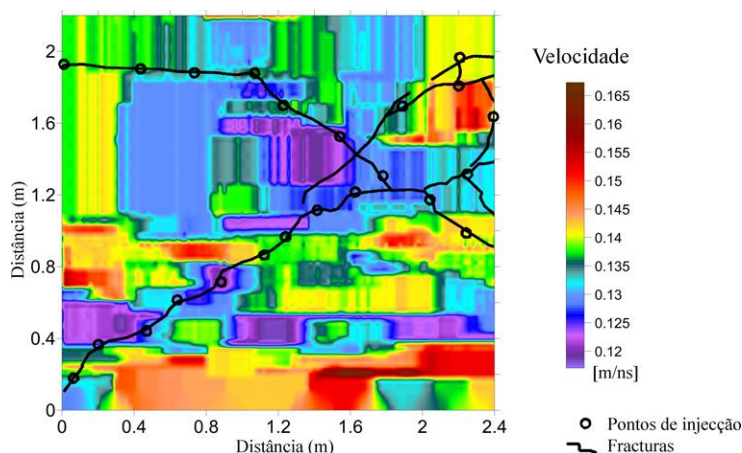
Figura 9: Distribuição de velocidades na parede
