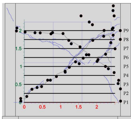
Figura 10: Perfis realizados entre ensaios mecânicos, mapeamento dos pontos de injeção da calda e de fracturas anteriores e posteriormente observadas.
