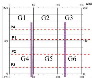
Figura 3: Perfis de georadar P1 a P4 (linhas a vermelho tracejado), de controlo de velocidade e projecção da posição das barras metálicas (linhas púrpura).
