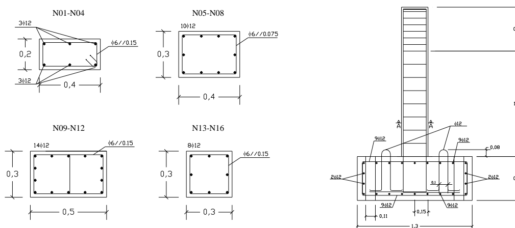
Figura 1. Pilares: geometria e pormenorização da armadura
