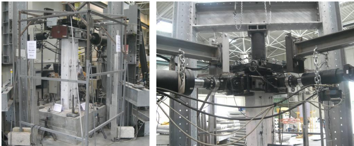
Figura 3. Esquema e vista do setup de ensaio no laboratório LESE
