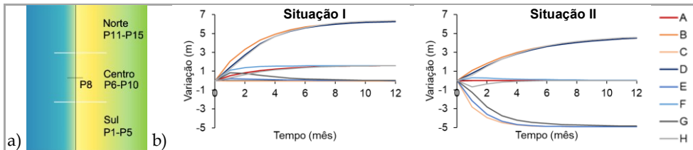
Figura 2. a) Domínio de cálculo; b) Evolução da variação da posição da linha de costa no perfil P8, para as duas situações de clima de agitação e os diferentes cenários de volume de barra (Tabela 1).
