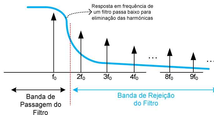
Figura 4 – Processo de filtragem de harmónicos
