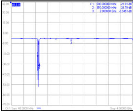
Figura 17 - S_{11} para o TMA de GSM900
