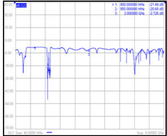
Figura 18 - S_{22} para o TMA de GSM900
