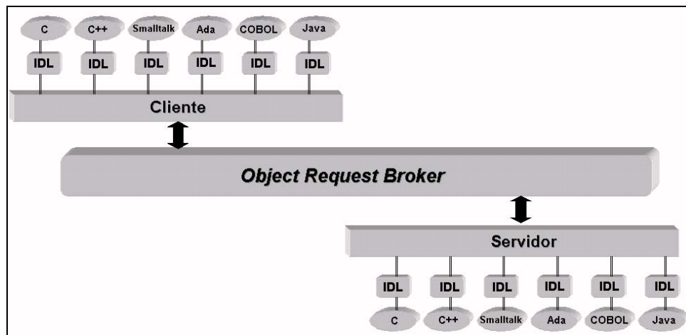
Figura 12 - Linguagem de Definição de Interfaces.
