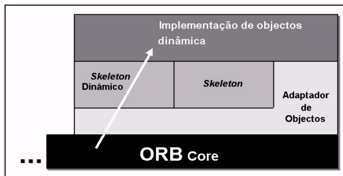
Figura 17 - Interface de Serviços Dinâmica.
