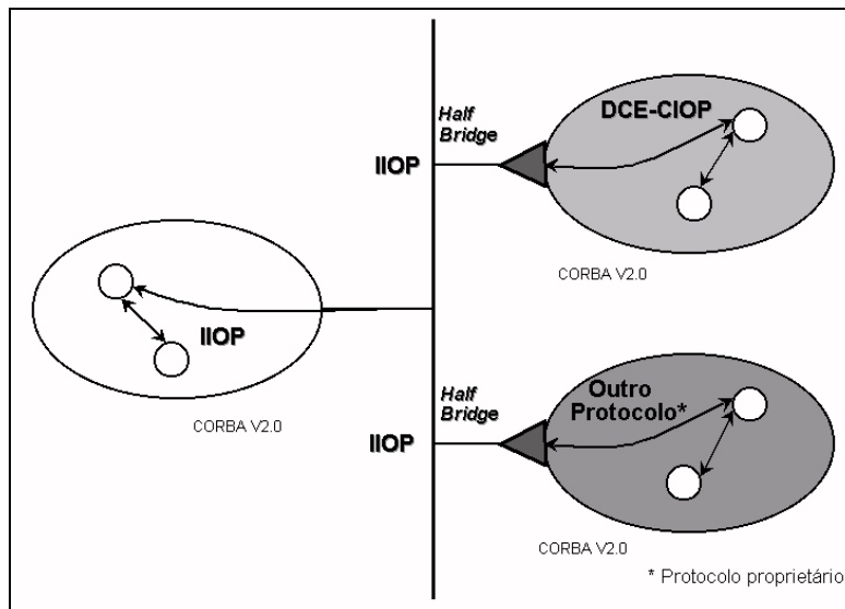
Figura 22 - Exemplos de interoperabilidade CORBA.
