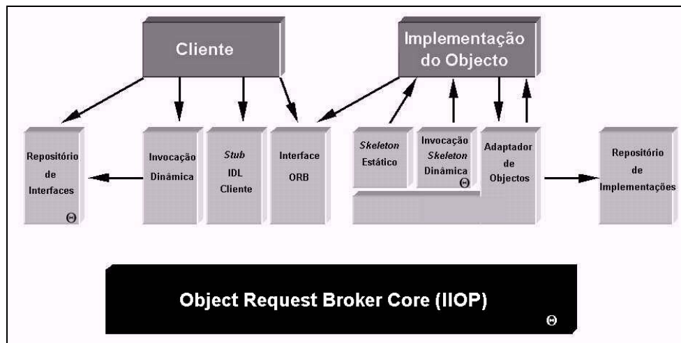
Figura 10 - Arquitectura do ORB.
