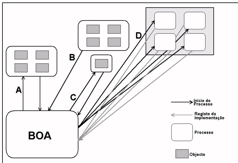
Figura 21 - Políticas de activação de implementações.
