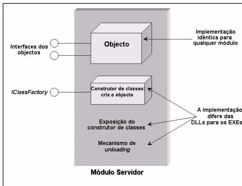
Figura 44 - Estrutura geral de um servidor DCOM.
