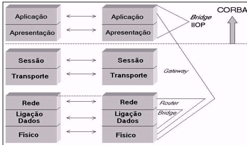
Figura 23 - IIOIP e bridges de rede.
