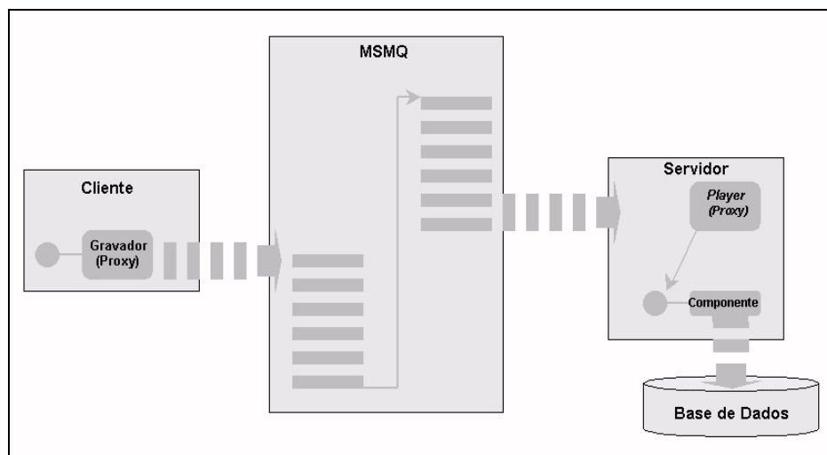
Figura 56 - Componentes em Fila.
