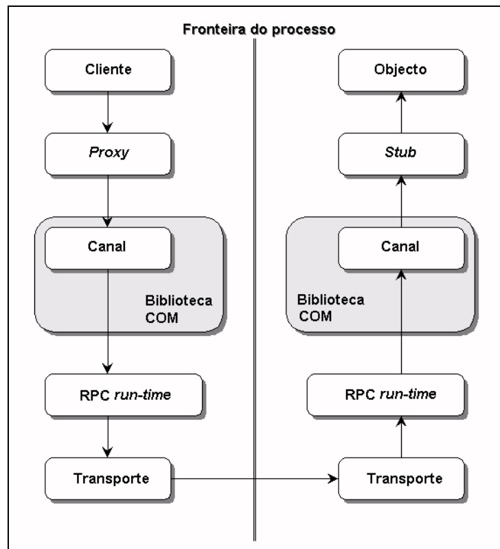
Figura 45 - Componentes da arquitectura distribuída DCOM.
