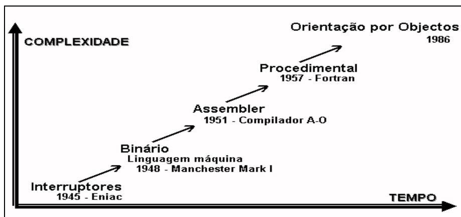
Figura 2 - Complexidade crescente.
