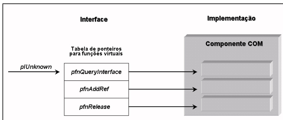
Figura 38 - Interface IUnknown .
