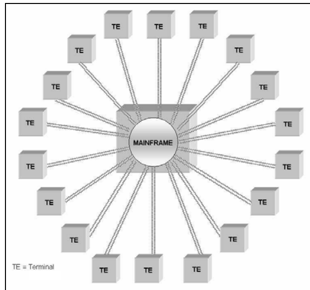
Figura 3 - Arquitectura centralizada.
