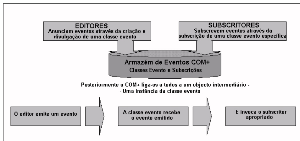
Figura 55 - Modelo de Eventos COM+.
