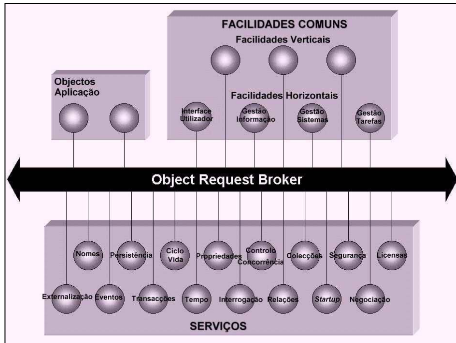
Figura 29 - Arquitectura de Gestão de Objectos.
