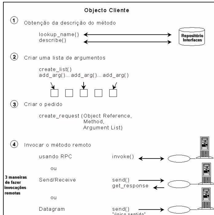
Figura 16 - Interface de Invocação Dinâmica.
