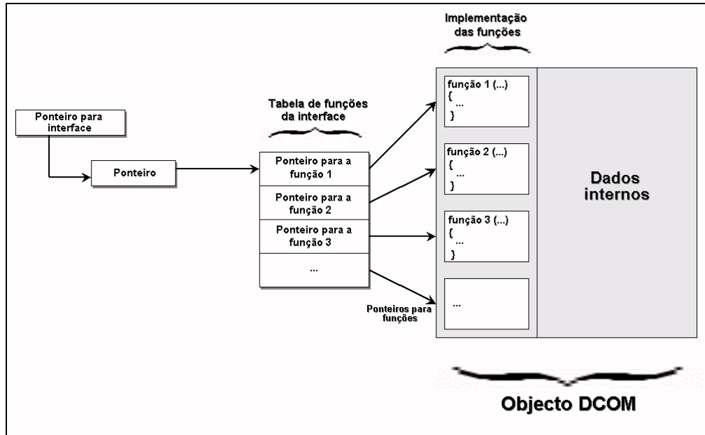
Figura 34 - Estrutura das interfaces.
