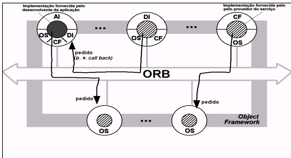
Figura 9 - Exemplo do fluxo de um pedido [OMG - 1997].
