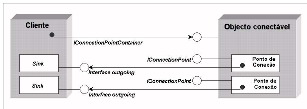
Figura 47 - Pontos de conexão.
