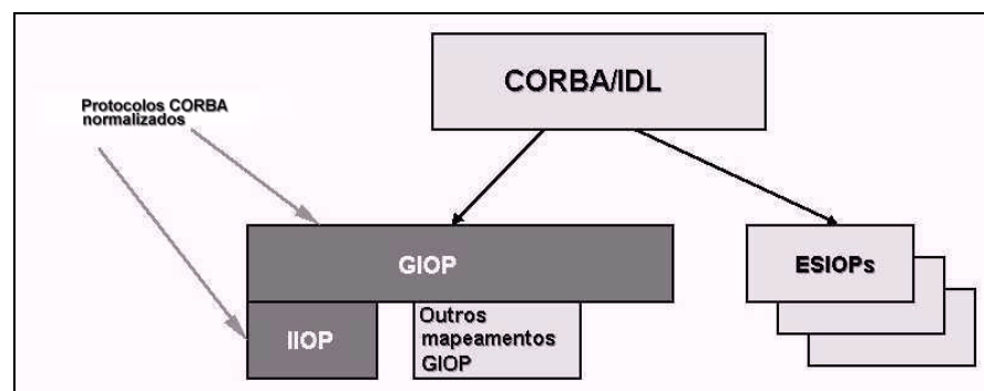
Figura 24 - Relação entre protocolos.
