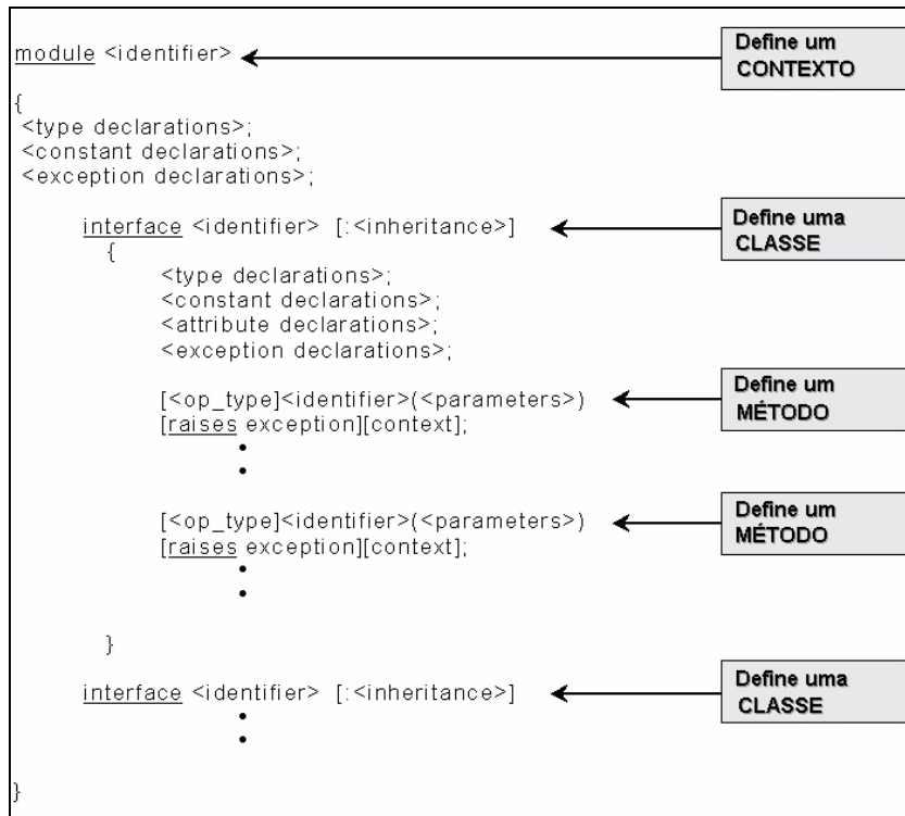
Figura 13 - Estrutura de um ficheiro IDL.
