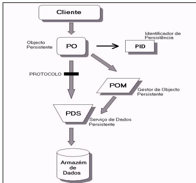
Figura 28 - Componentes principais do POS e suas iterações.
