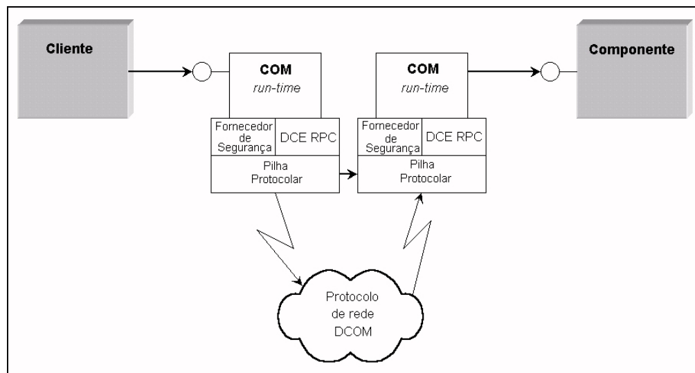
Figura 32 - Arquitectura DCOM - Comunicação entre componentes DCOM.
