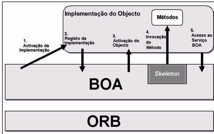
Figura 20 - Estrutura e operação do BOA.
