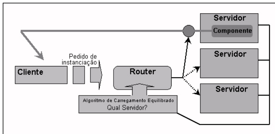
Figura 53 - Carregamento Equilibrado.
