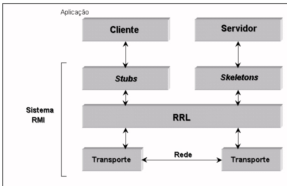
Figura 57 - Arquitectura JavaRMI.
