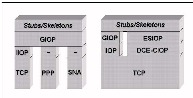
Figura 25 - Interoperabilidade CORBA.
