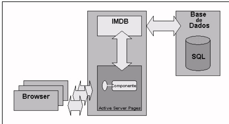
Figura 54 - IMDB COM+.
