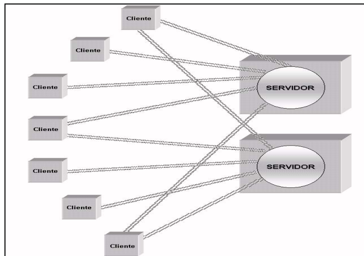
Figura 4 - Arquitectura cliente/servidor.
