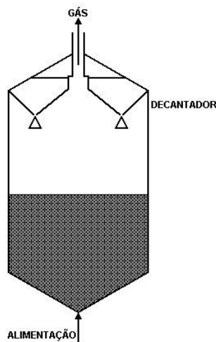
Figura 6- Representação esquemática de um reator UASB
