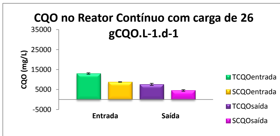
Figura 11- Valores de CQO médios à entrada e à saída no reator contínuo com uma carga de 26 g CQO.L -1 .d -1
