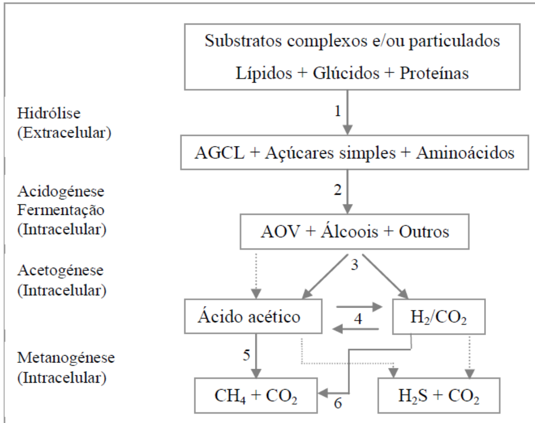
Figura 4- Representação esquemática das etapas constituintes da digestão anaeróbia, adaptada de Demirel e Scherer (2008), O’Flaherty et al (2006) e Pavlostathis e Giraldo-Gomez (1991). Os números representam os grupos microbiológicos envolvidos (ver Legenda)
