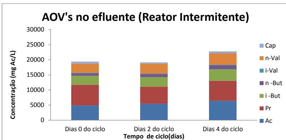
Figura 18- Ácidos orgânicos voláteis formados no reator intermitente nos dias 0, 2 e 4 do ciclo (carga de 22,9 \text{ g CQO.L}^{-1}.\text{d}^{-1} )
