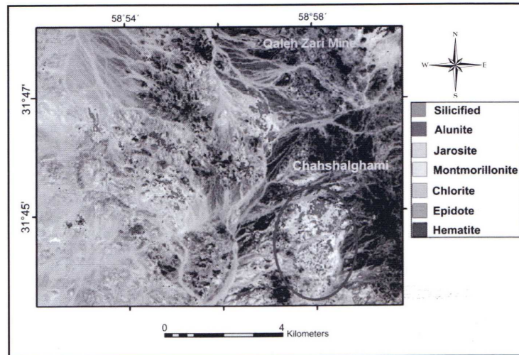
شکل ۶- هاله اصلی و انواع کانیهای دگرسانی در منطقه چاهشلغمی (کریمپور، ۱۳۸۴).
