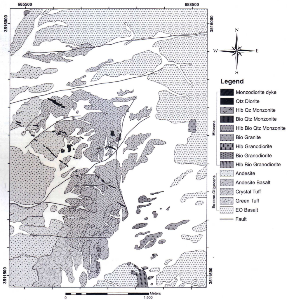
شکل ۲- نقشه زمین‌شناسی ۱:۵۰۰۰ چاه‌شلمی (ارجمندزاده و همکاران، ۲۰۱۱).
