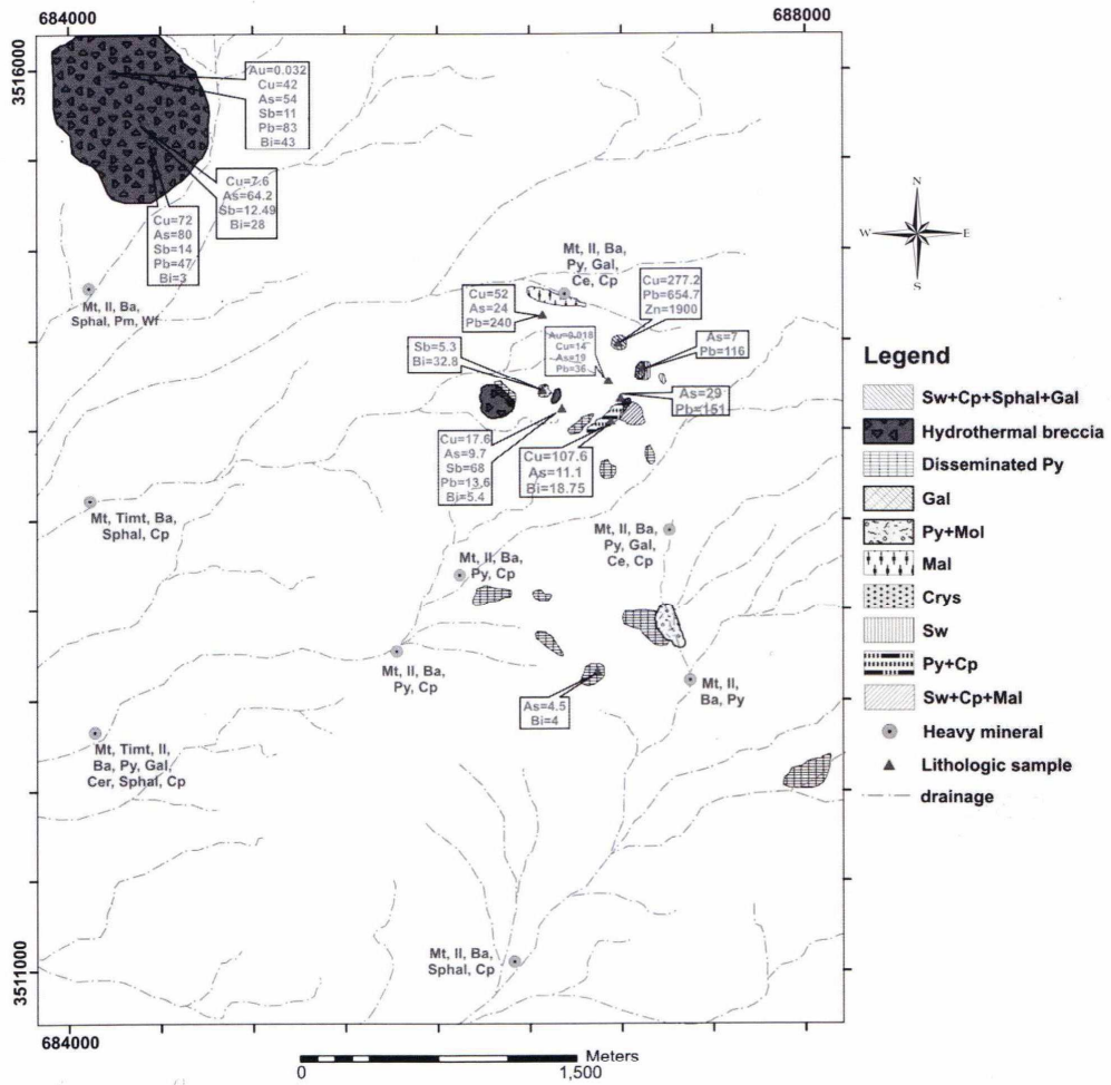
شکل ۸- نقشه کانی‌سازی و ژئوشیمیایی منطقه چاه شلمغی (ارجمندزاده و همکاران، ۲۰۱۱). علائم اختصاری شامل موارد زیر هستند: Sw: Stockwork, Cp: Chalcopyrite, Sphal: Sphalerite, Gal: Galena, Py: Pyrite, Mol: Molibdenite, Mal: Malakite, Crys: Chrysocolla, Mt: Magnetite, Timt: Titanomagnetite, Il: Ilmenite, Ba: Barite, Cer: Cerussite, Wf: Wulfenite
