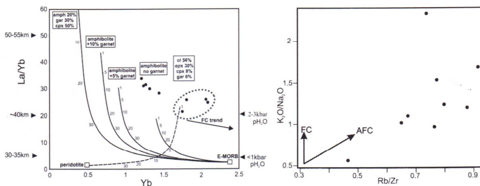
شکل ۱-۱ و ۱۱-۲ - نمایش توده‌های نفوذی چاه‌شلمگی در نمودارهای La/Yb - Yb و Rb/Zr در مقابل K_2O/Na_2O
