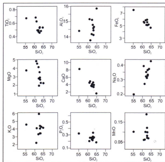
شکل ۹- نمایش توده‌های نفوذی چاه‌شغمی در نمودارهای هارکر
