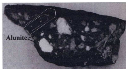
شکل ۷- بلورهای اولیه آلونیت در زون کوارتز- آلونیت
