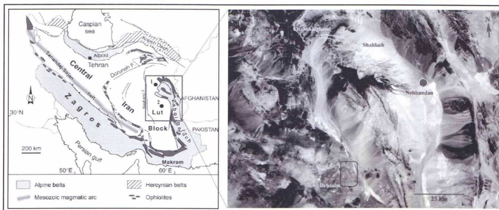
شکل ۱- نقشه زمین‌شناسی ایران (بربریان و کینگ، ۱۹۸۱) و موقعیت توده‌های نفوذی دهسلم و چاه‌شلمگی در تصویر ماهواره‌ای
