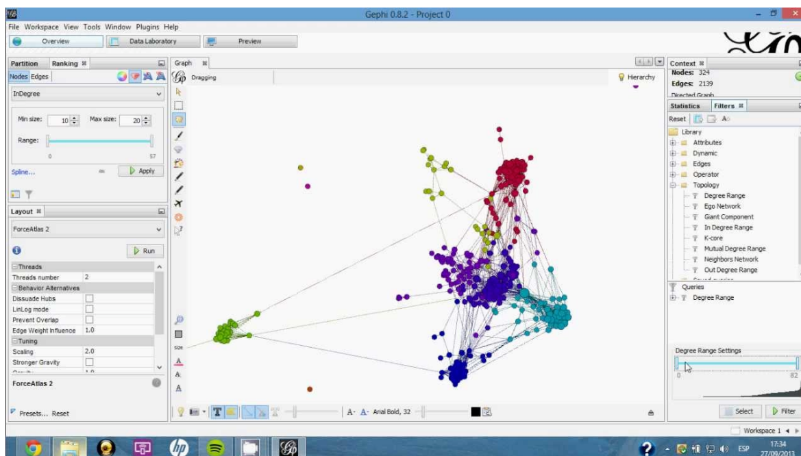
Figura 5 Gephi
