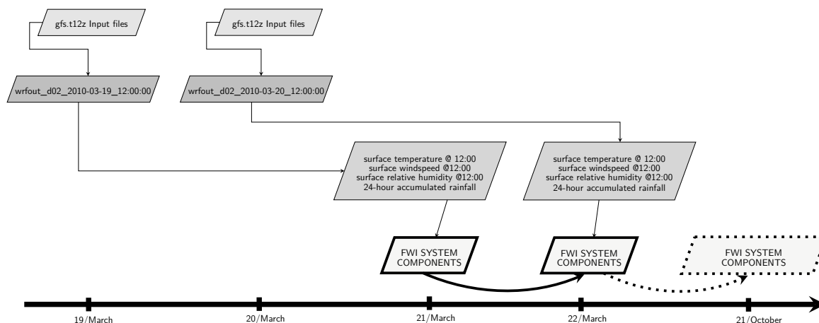
Figura 7.9: Esquematização dos procedimentos inerentes ao acoplamento ad hoc do modelo FWI canadiano com os resultados das previsões WRF, a 48 horas.
